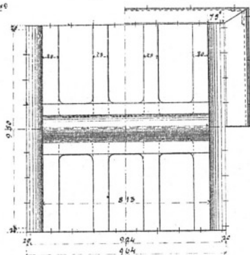
Планъ нижняго балансира Видъ сверху
