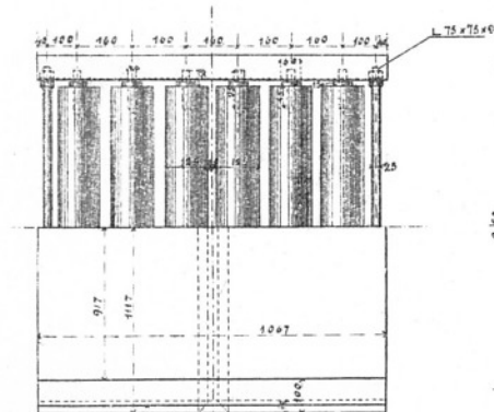
Планъ катковъ
