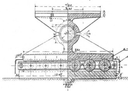
Боковой видъ Разрѣзъ
