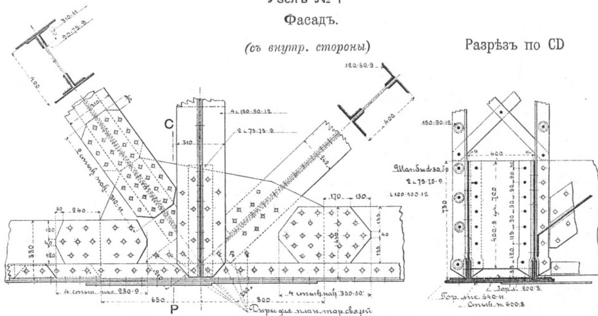
Узелъ № 1
