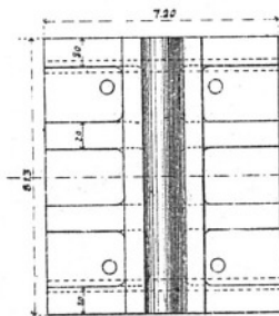
Планъ верхняго балансира Видъ снизу
