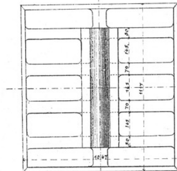
Планъ нижняго балансира
