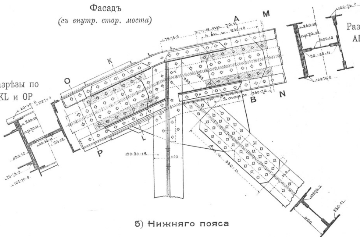
Узелъ № 1
