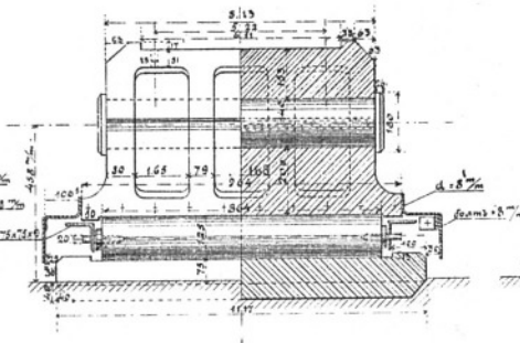
Боковой видъ Разрѣзъ
